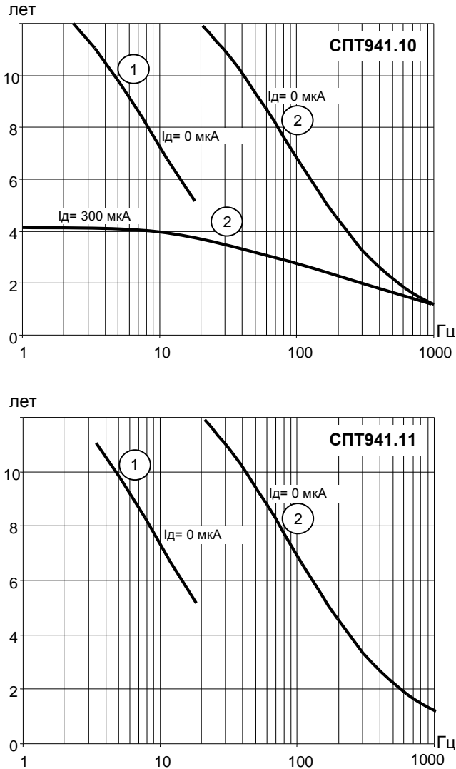
Рисунок 2.1 – Зависимость ресурса батареи (лет) от частоты входных импульсов (Гц) и суммарного среднего тока потребления преобразователей объема I_d .
