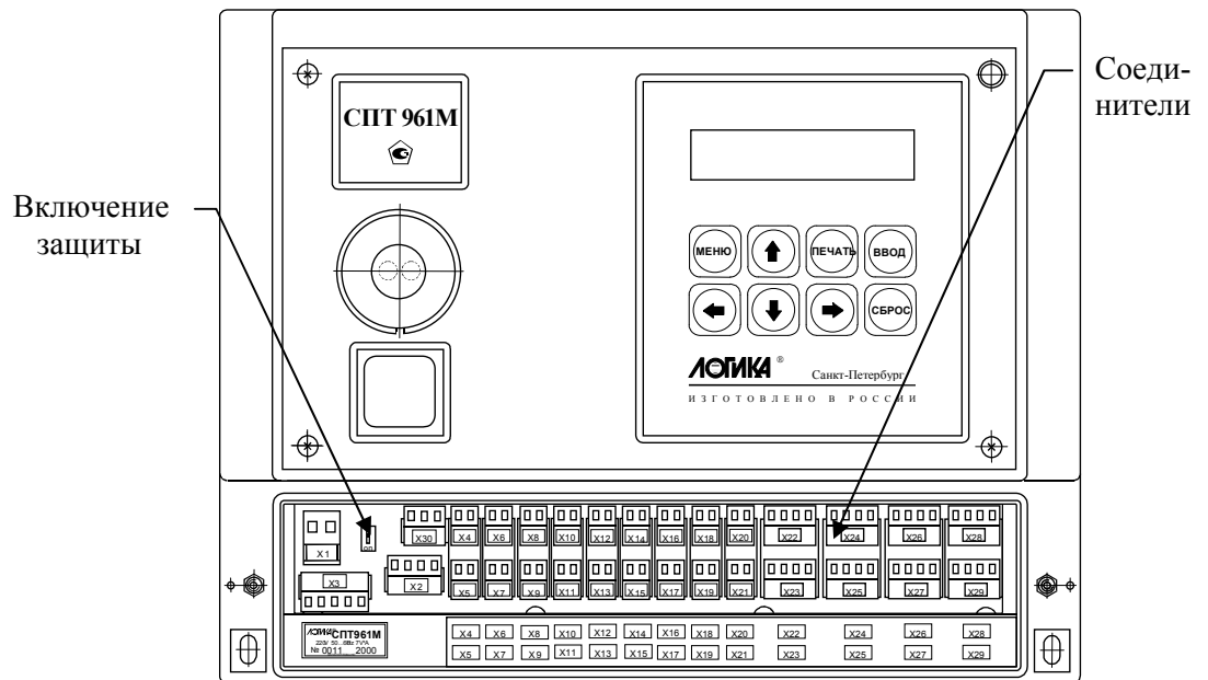
Рисунок 3.2 Тепловычислитель СПТ961М. Вид спереди
