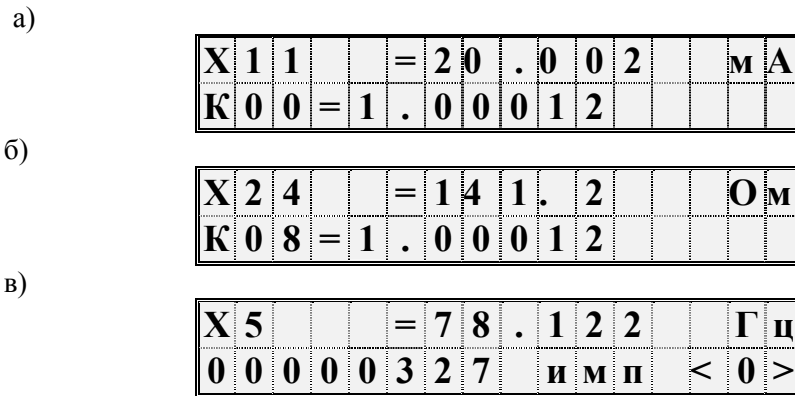
Рисунок 5.12 Табло прибора в режиме тестирования АВВ
